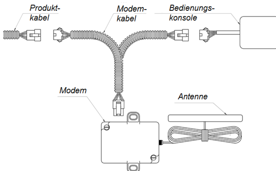
Abb. 2. Anschluss des Modems an die Produkte der Baureihe BINAR-5-Compact, BINAR-5S und PLANAR.
